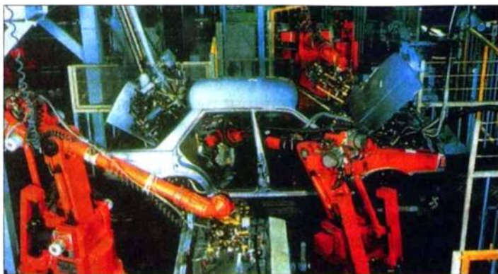
Автоматизированный конвейер на автомобильном заводе «Хонда»
